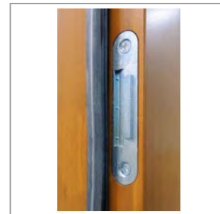
AUSHEBESICHERUNGEN 2 Stück an Bandseite montiert Stahl, Farbe Topzink
